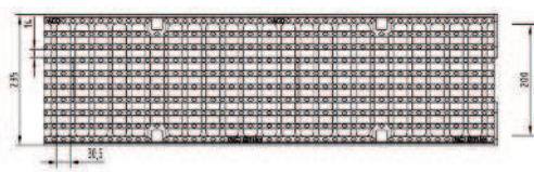
Grille caillebotis fonte
