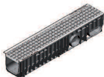
150 , Caniveau type 01 avec caillebotis mailles 30 x 30, galva, classe B 125, monté
