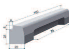
T3 Avaloir Non traversant 1 m
