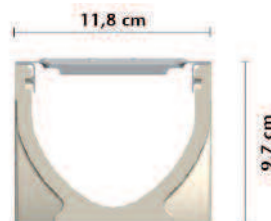
Section du caniveau 100% libre sans barette
