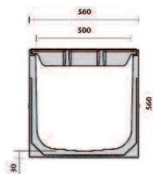
Caniveau S500
