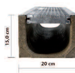
Section du caniveau 100% utile
