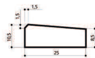
CS2 réduit
