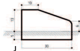
SERIE I4
