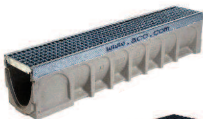
Multidrain 150 avec grille caillebotis
