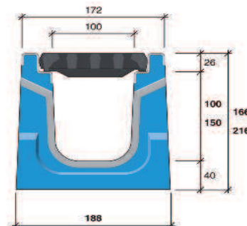
Caniveau RI 100
