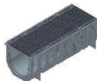
300 , Caniveau type 010 avec GUGI caillebotis fonte, mailles 20 x 30, noire, classe C 250
