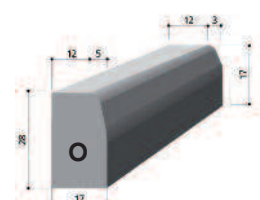
T2 Biais pressée Gauche ou droite
