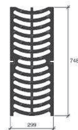
Grille 7530 BAN D400
