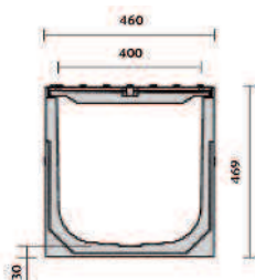
Caniveau S400
