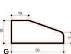
SERIE I3
