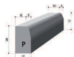
T3 Biais Gauche ou droite
