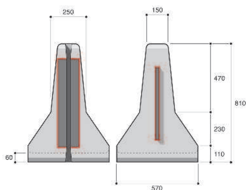
Glissière EGS
